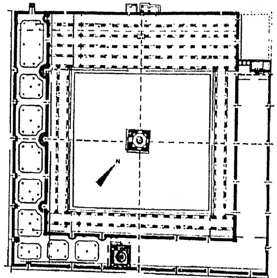
الشكل ٢٢-٨، خارطة بناء مسجد ابن طولون (بناء ذو سقف مُعمد) القاهرة (٨٧٦ - ٨٧٩).
